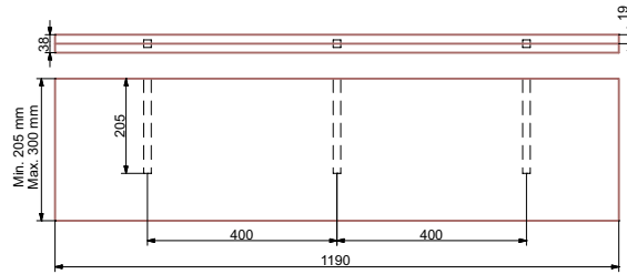
Pour support invisible LHTABIN For concealed bracket LHTABIN
