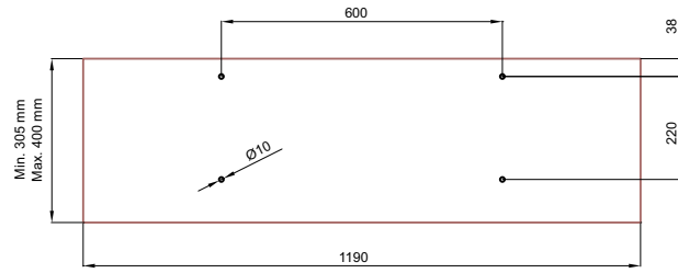
Pour support tablette 300 mm LHTAB30B et LTTAB30B Pour support pendu côté / plié LHBPTABB et LTBPTABB For 300-mm shelf brackets LHTAB30B and LTTAB30B For shelf + clothes rail brackets LHBPTABB and LTBPTABB
