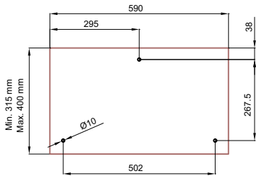
Pour support tablette T LHTABTB et LTTABTB For T-brackets LHTABTB and LTTABTB
