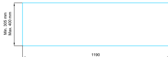
Pour support tablette 300 mm LHTAB30V et LTTAB30V Pour support pendu côté / plié LHTABTV et LTBPTABV For 300-mm shelf brackets LHTAB30V and LTTAB30V For shelf + clothes rail brackets LHTABTV and LTBPTABV
