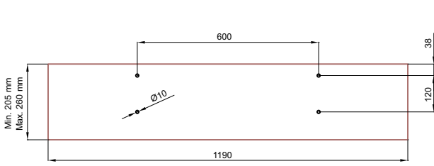
Pour support tablette 200 mm LHTAB20B et LTTAB20B For 200-mm shelf brackets LHTAB20B and LTTAB20B
